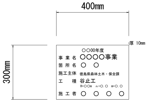
図1 銘板の寸法及び記載事項
